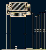
Vertikalschnitt Futter (RF)
