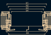
2-flügelig gefälzte Türen
