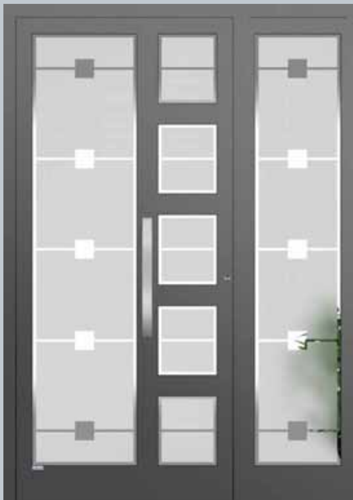
T 130 verschweiß , DB 703 dunkelgrau matt, Glas G 01 (Float teilmattiert), Griff 1704 Edelstahl
