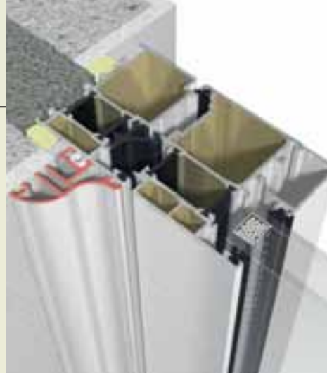
Wandanschlussprofil für den Außenbereich, hier am Beispiel einer GRAUTE-Therm-80-Haustür
