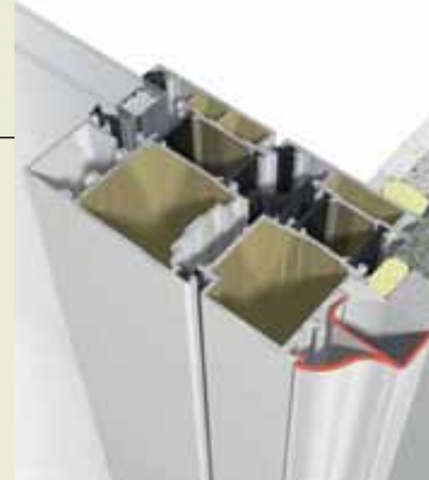
Wandanschlussprofil für den Innenbereich
