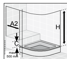
Abb. 5 Runddusche mit Frontver- längerung und Ausschnitt Höhenänderung möglich: Runddusche-Classic Kunststoffglas Breitenänderung möglich: Classic, Palladium de Luxe, Palladium 4-teilig, Sequenz und Glass5 Evolution
