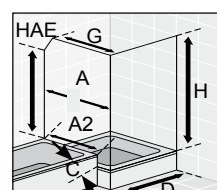
Abb. 20 Tür mit Seitenwand/Aus- schnitt/Schrägschnitt auf Badewanne möglich mit: Palladium, Palladium de Luxe, Sequenz, Glass5 Evolution und Classic
