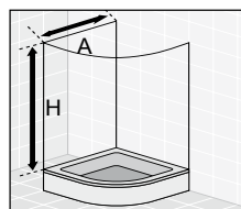
Abb. 2 Runddusche mit Seitenwand gleiche Höhe Höhenänderung möglich: Runddusche-Classic Kunststoffglas Breitenänderung der Seitenwand möglich: Classic, Palladium de Luxe
