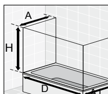
Abb. 26 Badewannenaufsatz mit 2 SW gleiche Höhe möglich mit: Schiebetür BSC
