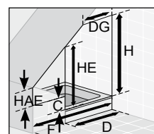
Abb. 15 Tür mit Schrägschnitt und verkürzter Frontwand möglich mit: Palladium und Palladium de Luxe
