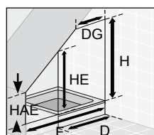
Abb. 14 Tür mit Schrägschnitt und Frontwand möglich mit: Palladium und Palladium de Luxe
