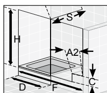
Abb. 11 Tür mit Frontwand u. Stabilisator Ausschnitt möglich, alle Modelle. Stabilisator ab Frontbreite von 400 mm erforderlich, außer Royalux Design und Royalux Design Vital
