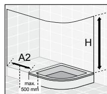
Abb. 4 Runddusche mit Frontver- längerung Höhenänderung möglich: Runddusche-Classic Kunststoffglas Breitenänderung möglich: Classic, Palladium de Luxe, Palladium 4-teilig, Sequenz und Glass5 Evolution
