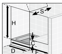
Abb. 12 Tür mit verkürzter Frontwand u. Stabilisator alle Modelle. Stabilisator ab Frontbreite von 400 mm erfor- derlich, außer Royalux Design und Royalux Design Vital
