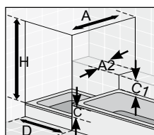
Abb. 21 Tür mit verkürzter Seitenwand und Ausschnitt möglich mit: Palladium, Palladium de Luxe, Sequenz, Glass5 Evolution und Classic
