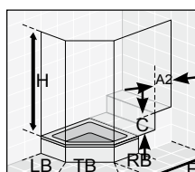
Abb. 33 Fünfeckdusche mit Frontverlängerung und Ausschnitt möglich mit: Palladium de Luxe, Sequenz und Glass5 Evolution
