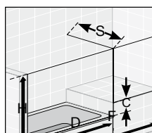
Abb. 28 Badewannenaufsatz mit verkürzter Frontwand möglich mit: Schiebetür BSC
