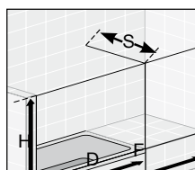
Abb. 27 Badewannenaufsatz mit Frontwand gleiche Höhe möglich mit: Schiebetür BSC
