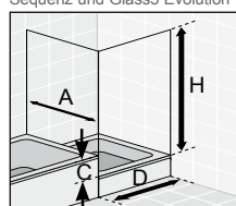
Abb. 9 Tür mit verkürzter SW alle Modelle
