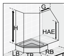
Abb. 34 Fünfeckdusche mit Frontverlängerung und Schrägschnitt möglich mit: Palladium de Luxe, Sequenz und Glass5 Evolution
