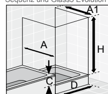
Abb. 10 Eckeinstieg mit verkürzter SW oder Tür mit SW gleiche Höhe und verkürzter SW möglich mit: Classic und Palladium
