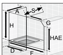
Abb. 13 Eckeinstieg mit FW o. Tür mit SW gleiche Höhe und FW u. Stabilisator möglich mit: Classic und Palladium
