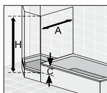
Abb. 31 Fünfeckdusche mit verkürzter Seitenwand möglich mit: Palladium de Luxe
