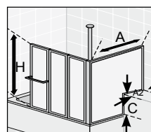
Abb. 29 BTT mit Seitenwand/Ausschnitt kein Schrägschnitt machbar!
