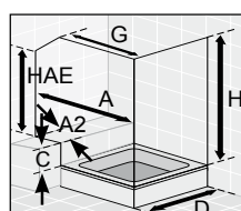
Abb. 19 Tür mit Seitenwand/Aus- schnitt/Schrägschnitt möglich mit: Palladium, Palladium de Luxe, Sequenz, Glass5 Evolution und Classic
