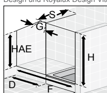
Abb. 16 Tür mit Frontwand/Schräg- schnitt u. Stabilisator alle Modelle außer Royalux Design und Royalux Design Vital Design
