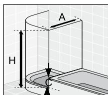
Abb. 3 Runddusche mit verkürzter Seitenwand Höhenänderung möglich: Runddusche-Classic Kunststoffglas Breitenänderung der Seitenwand möglich: Classic, Palladium de Luxe
